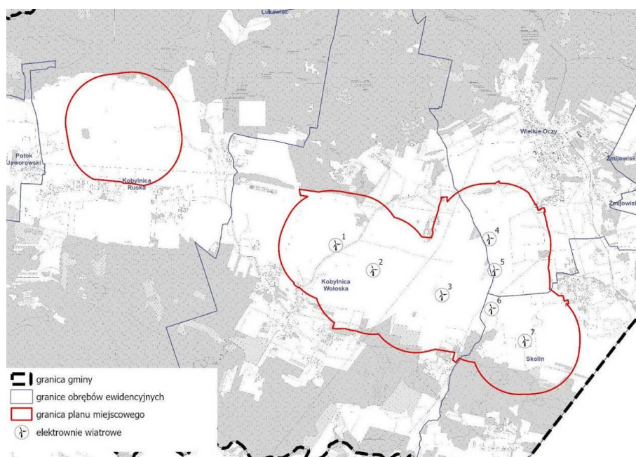
Rysunek 31. Projektowana lokalizacja elektrowni wiatrowych (źródło: opracowanie własne na podstawie projektu mpzp)
