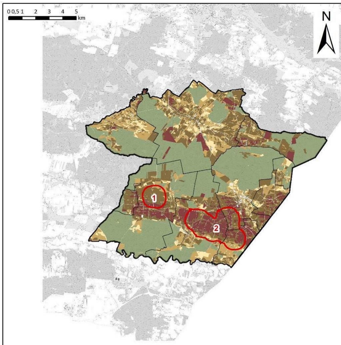
Rysunek 8. Gleby na terenie gminy (źródło: opracowanie własne na podstawie danych EGiB)
