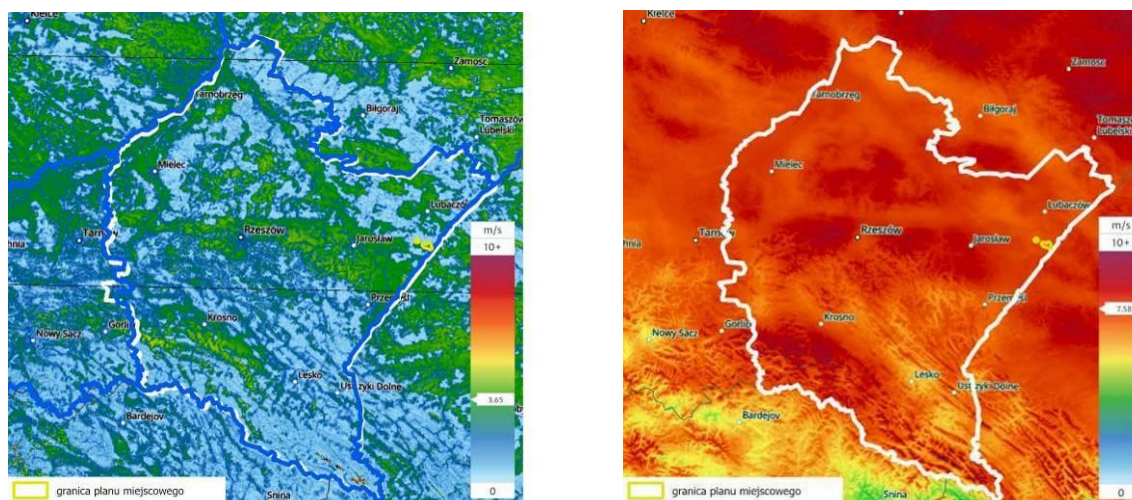
Rysunek 29. Obszar opracowania na tle mapy średniej prędkości wiatru na wysokości 10 m (po lewej) i 200 m (po prawej) (źródło: opracowanie własne na podstawie Globalnego Atlasu Wiatru)
