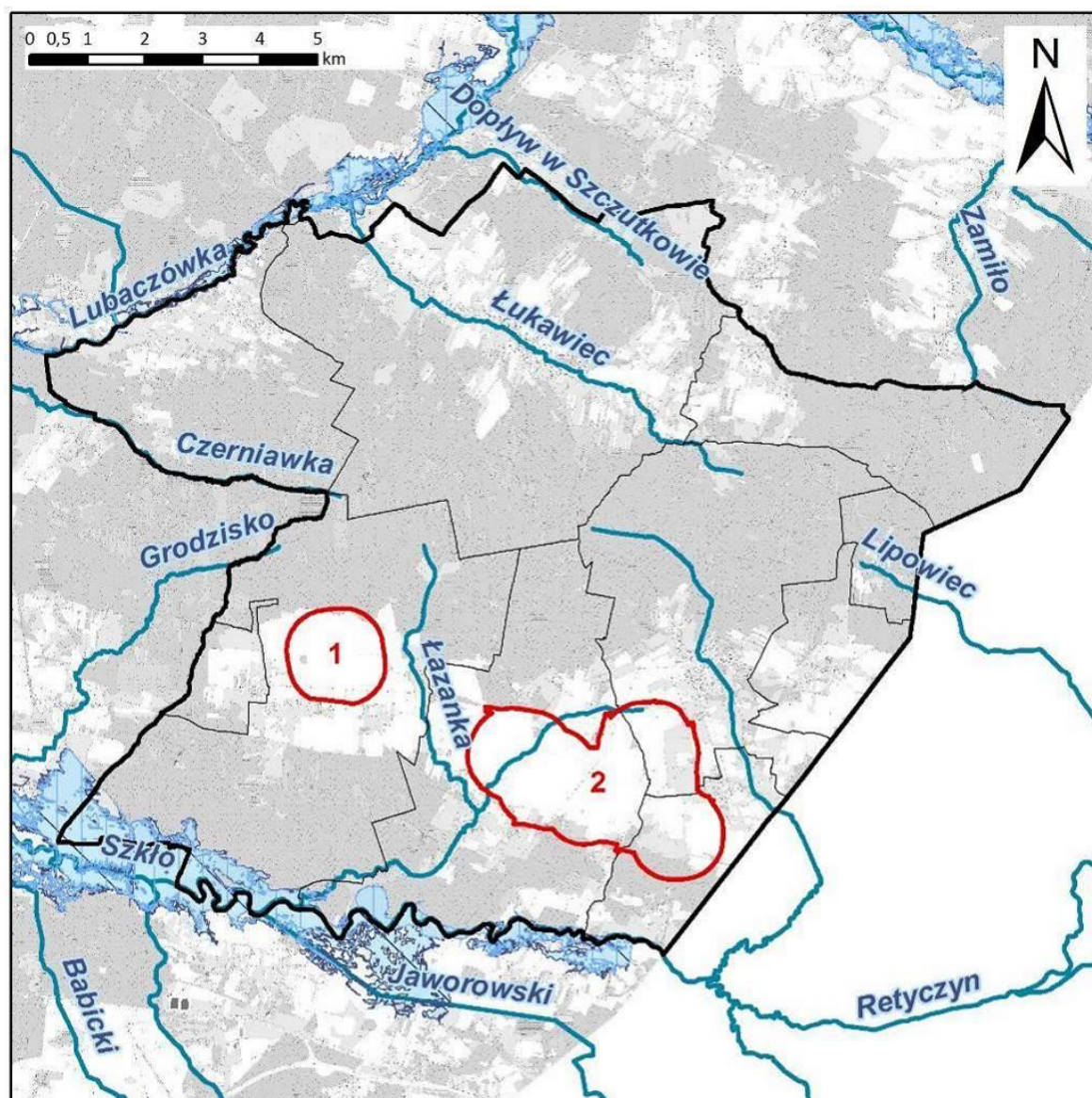
Rysunek 24. Zagrożenie powodziowe w Gminie Wielkie Oczy (źródło: opracowanie własne na podstawie danych przestrzennych PGW Wody Polskie)
