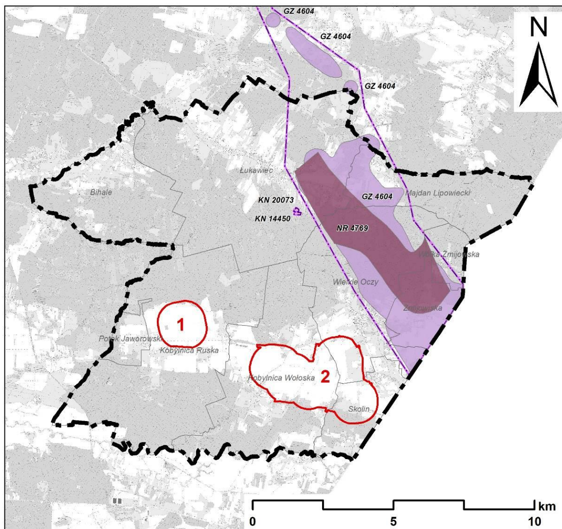
Rysunek 7. Udokumentowane złoża kopalin, obszary i tereny górnicze na terenie Gminy Wielkie Oczy (źródło: opracowanie własne na podstawie warstw tematycznych PIG-PIB: Surowce – złoża kopalin, obszary górnicze, tereny górnicze)
