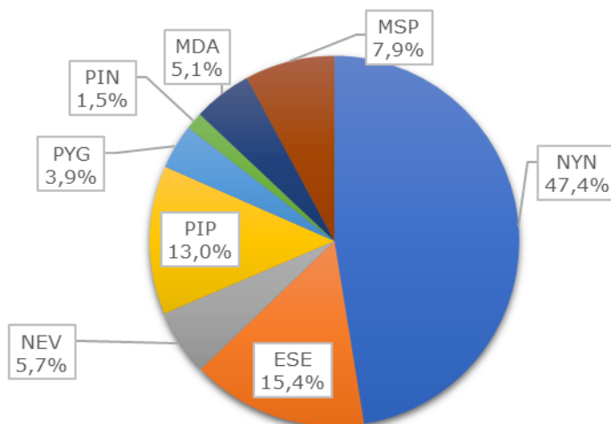
Rysunek 16. Procentowy udział wszystkich gatunków nietoperzy zarejestrowanych na transektach i w punktach nasłuchowych w granicach powierzchni badawczej (grunty inwestycyjne i bufor) (źródło: Raport z rocznej realizacji przedrealizacyjnego monitoringu Chiropterofauny obszaru projektowanej Farmy Wiatrowej Wielkie Oczy, 2025)
