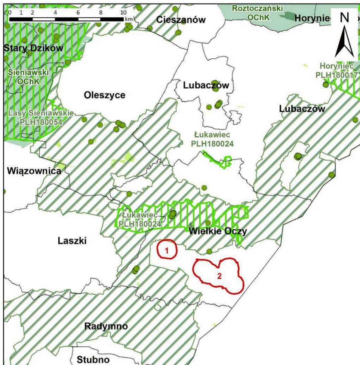
Rysunek 21. Korytarze ekologiczne łączące obszary Natura 2000 na terenie gminy (źródło: opracowanie własne na podstawie danych GDOŚ)
